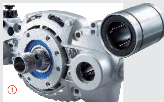
① Robuste : utilisation de roulement large et protection maximale contre les poussières grâce à la ventilation de la zone de travail et à la construction renforcée.
