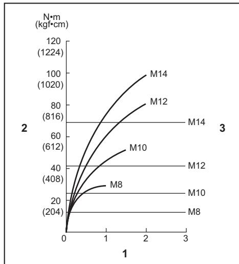
1. Tiempo de apriete (segundo) 2. Par de apriete 3. Par de apriete apropiado correspondiente a cada diámetro de perno
