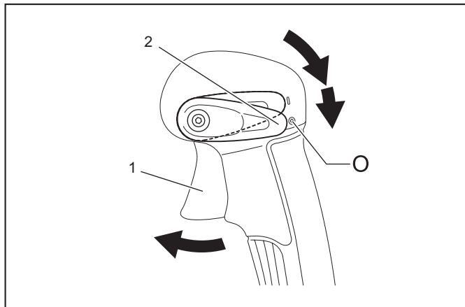
► 1. Gasabzug 2. Drehzahlsteuerhebel
