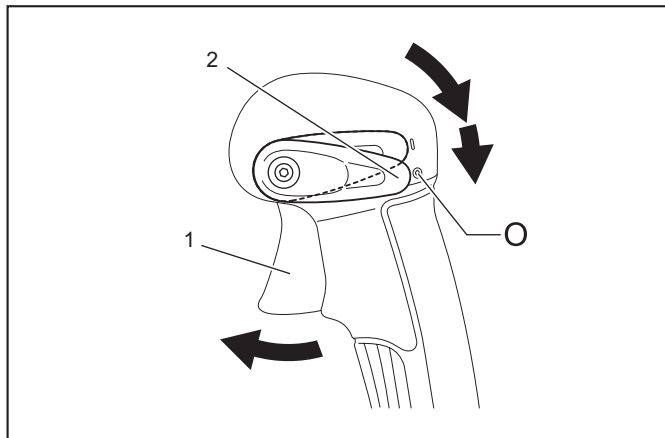
► 1. Σκανδάλη στραγγαλισμού 2. Μοχλός ελέγχου διακοπής
