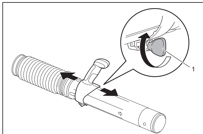
► 1. Parafuso
