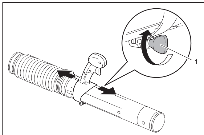
► 1. Schraube
