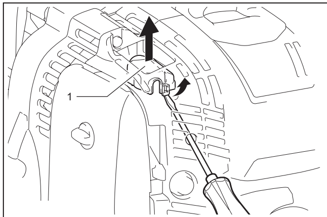
► 1. Tampa do carburador
