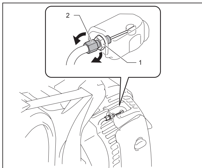
► 1. Befestigungsmutter 2. Seilzug-Einstellschraube
