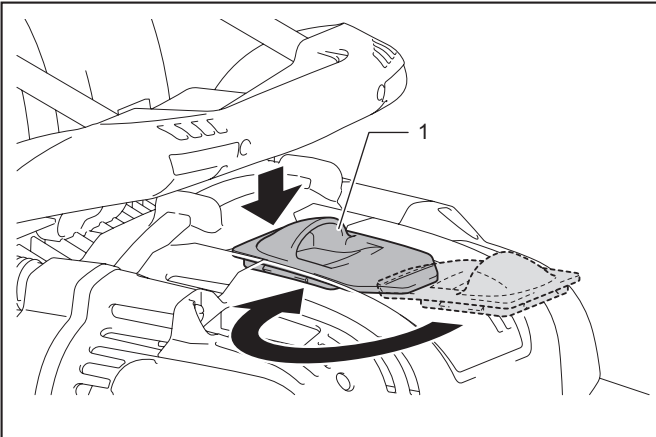
► 1. Buji kapağı
