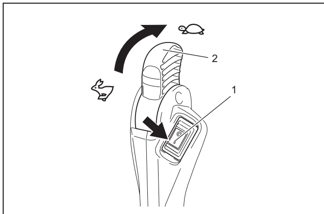
► 1. Stopschakelaar 2. Gashendel
