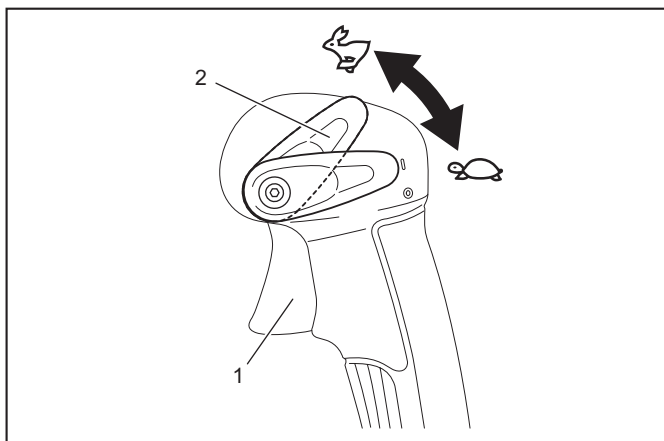
► 1. Gasspjældstrigger 2. Stopkontrolarm
