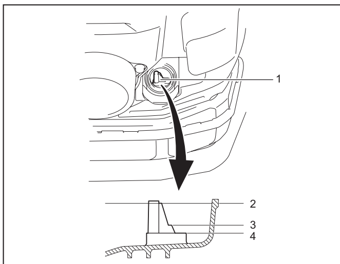
► 1. Medidor de nivel de aceite 2. Marca de límite superior 3. Nivel de 100 ml 4. Marca de límite inferior
