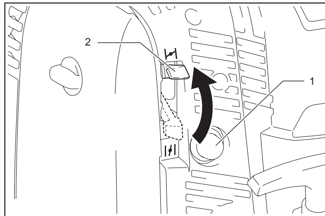
► 1. Αντλία προέγχυσης 2. Μοχλός τσοκ
