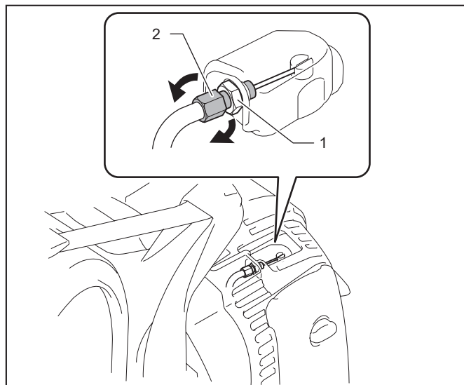
► 1. Fastgørmøtrik 2. Kabeljusteringsbolt
