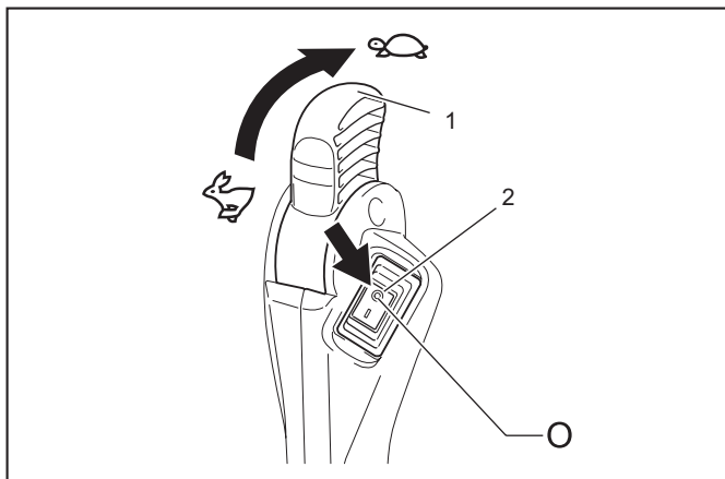
► 1. Gashåndtag 2. Stopknop
