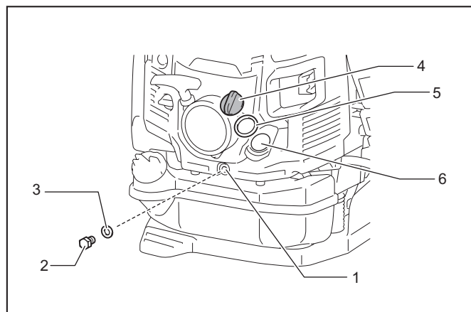
► 1. Afløbshul 2. Oliedrænbolt 3. Pakning (aluminiumspakningskive) 4. Oliehætte 5. Pakning på oliehatte 6. Olieåbning
