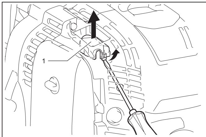
► 1. Κάλυμμα καρμπυρατέρ
