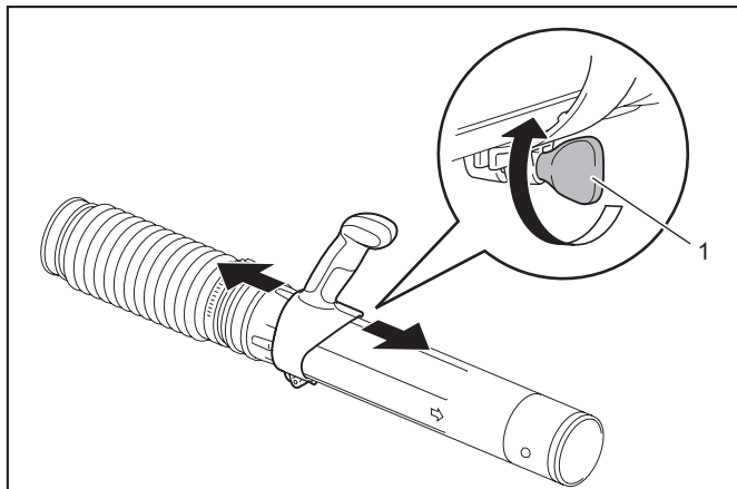
► 1. Tornillo
