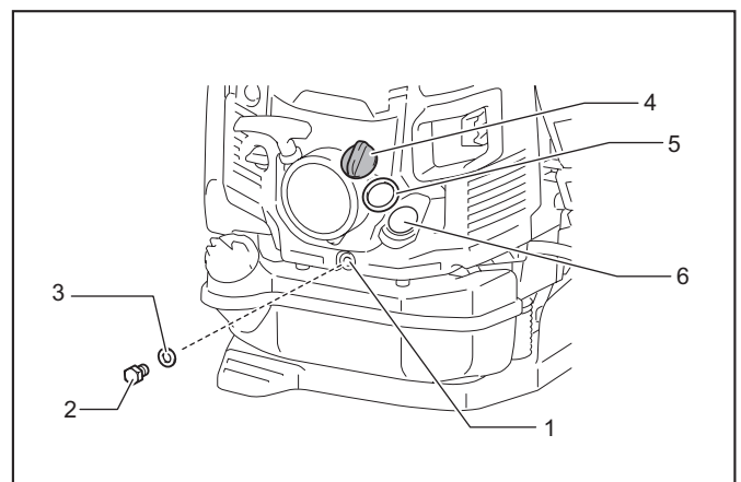
► 1. Ablassöffnung 2. Ölablassschraube 3. Dichtung (Aluminiumscheibe) 4. Öldeckel 5. Öldeckeldichtung 6. Ölöffnung
