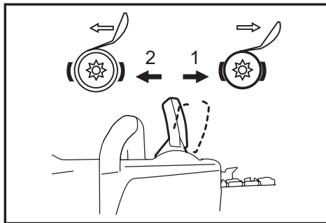
1. Ketipidur rakendatud 2. Ketipidur vabastatud
